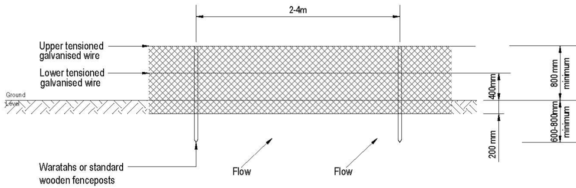
Elevation
